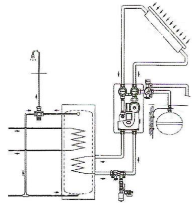
2. Ηλιοθερμικό σύστημα παραγωγής ζεστού νερού χρήσης
